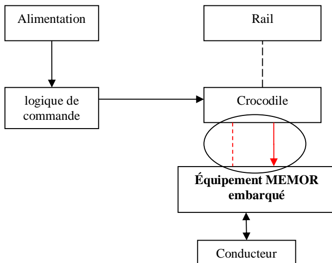
Figure 1 : Diagramme contextuel
